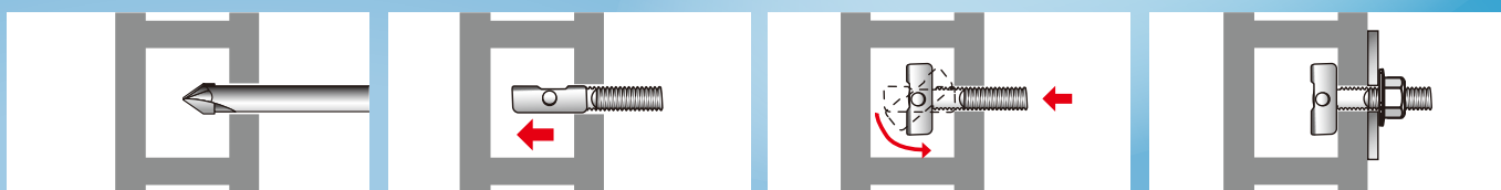
① アメラドリルで穿孔 ※裏面をご確認ください。
