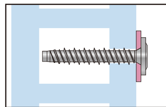
③施工完了 取付物を固定する
