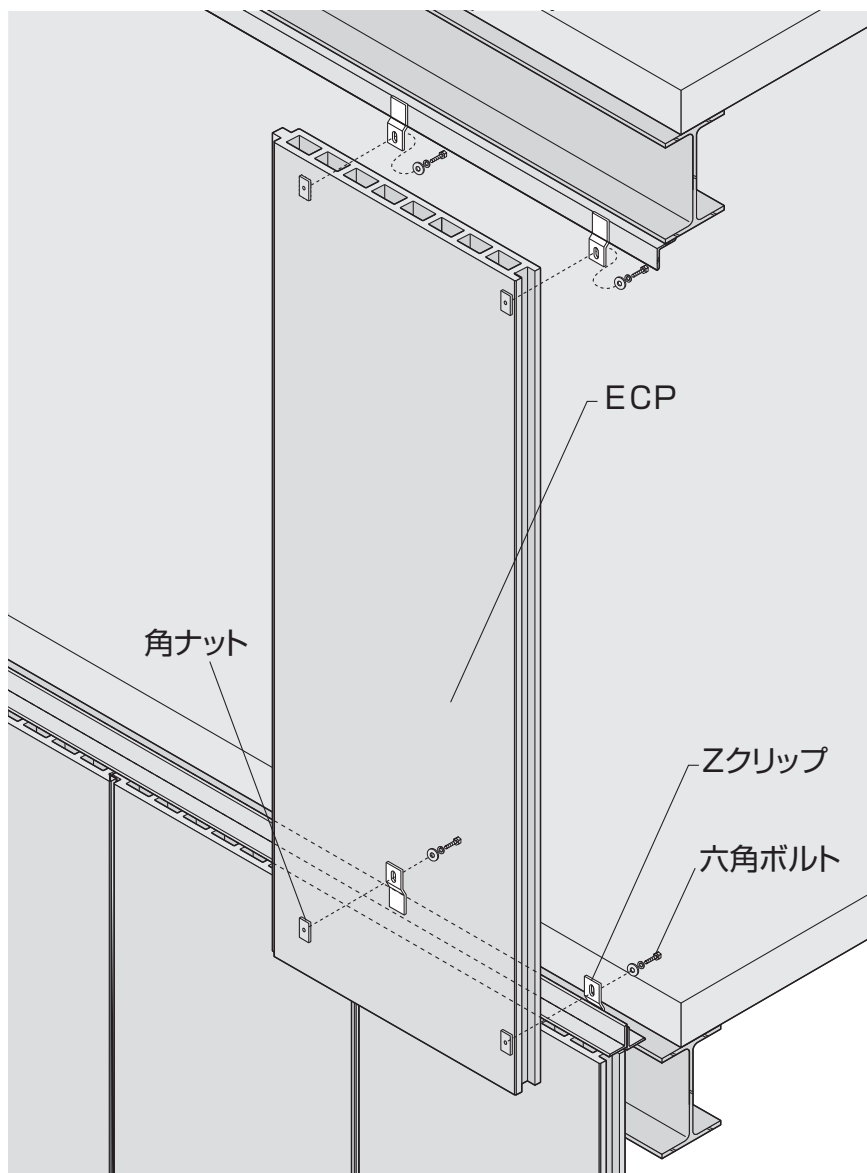
ECPの標準的な取付け方
