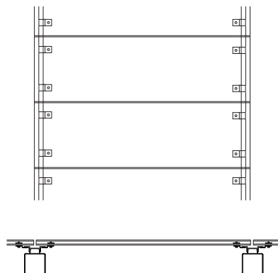
図 横張り工法
