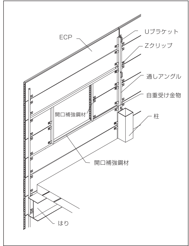
図1-2 横張り工法
