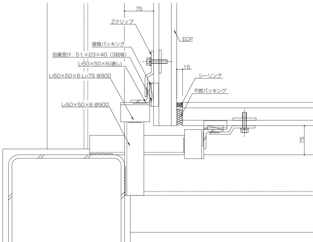
3-12 入隅コーナー部詳細図
