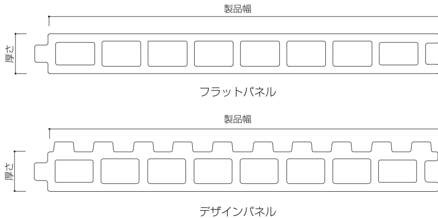
図2-2 形状の例
