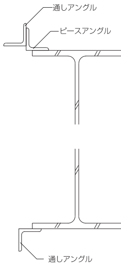
図4-13 縦張り工法中間部下地鋼材取付け状況
