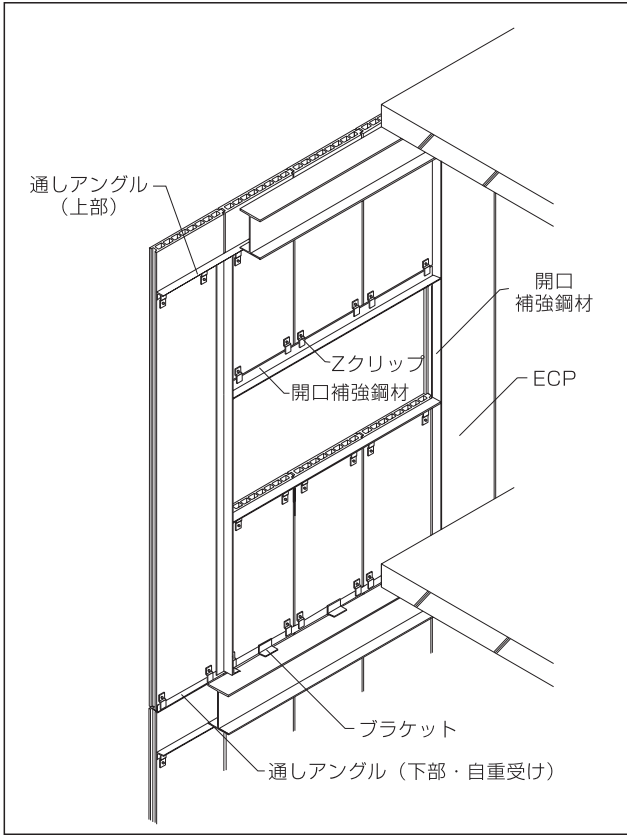
図1-1 縦張り工法
