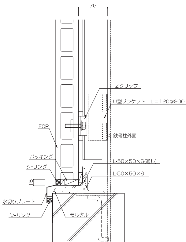
3-8 下部垂直断面詳細図
