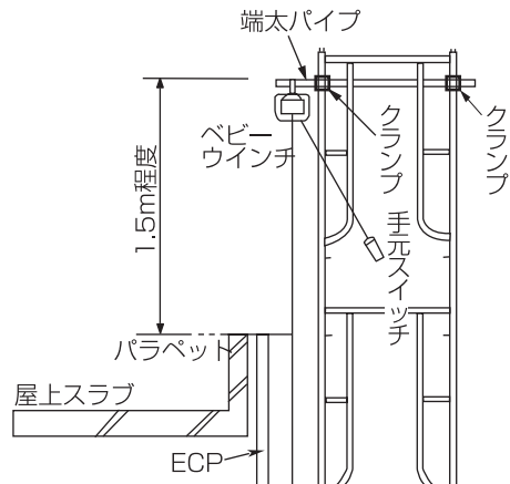
図3-3 足場
