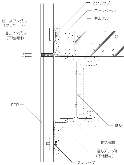
図4-6 縦張り工法中間部標準詳細図
