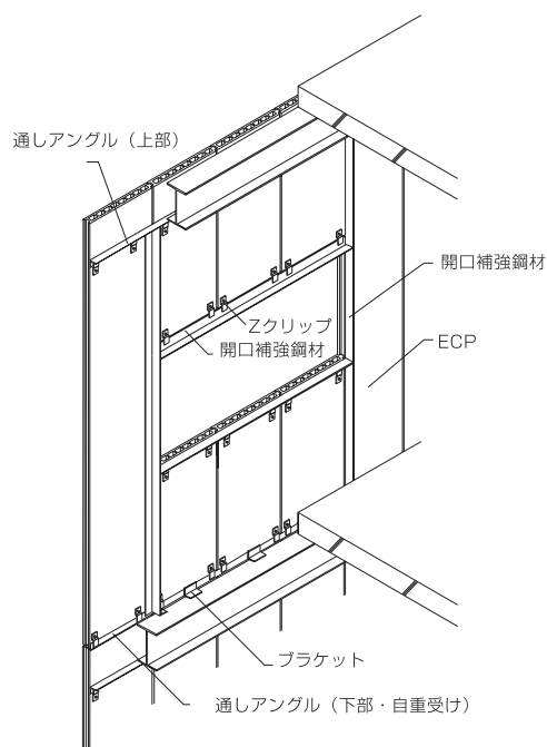
図4-1 縦張り工法
