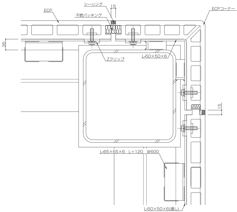
3-6 入隅コーナー部詳細図
