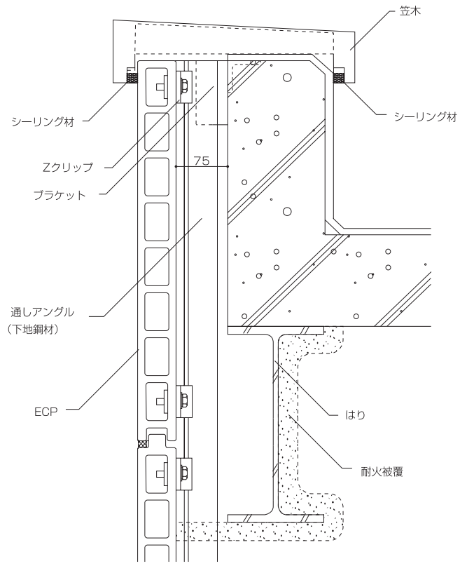
図4-11 横張り工法上部標準詳細図
