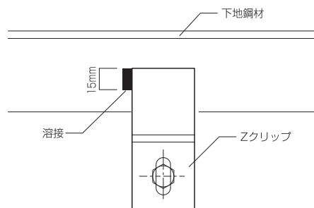
図4-15 Zクリップのかけり代
