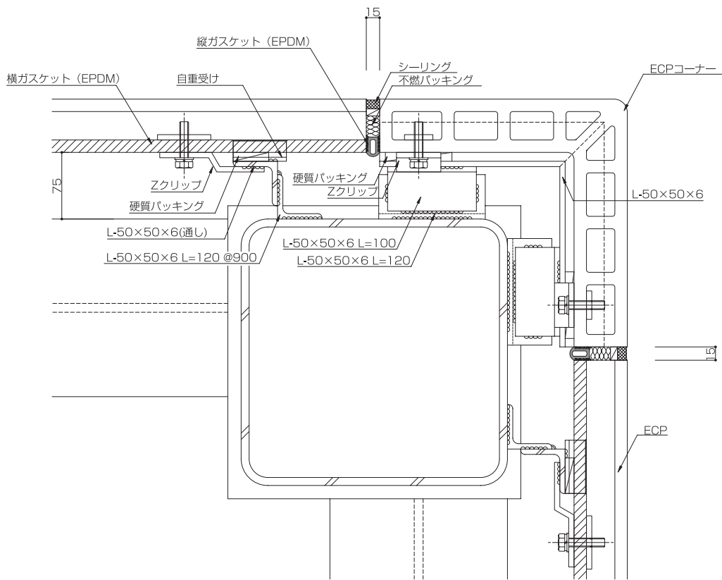
出隅コーナー部詳細図
