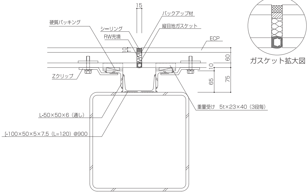
水平断面図
