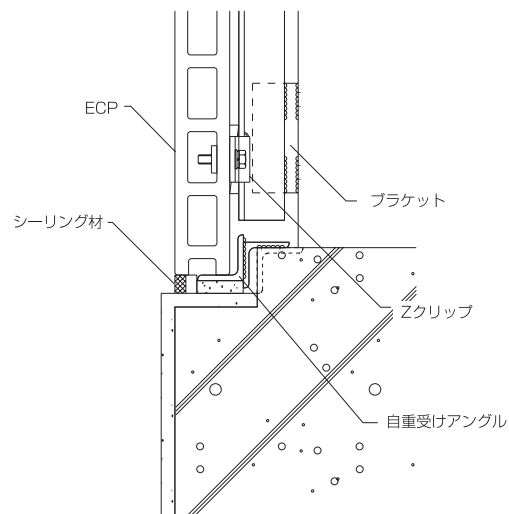
図4-9 横張り工法下部標準詳細図
