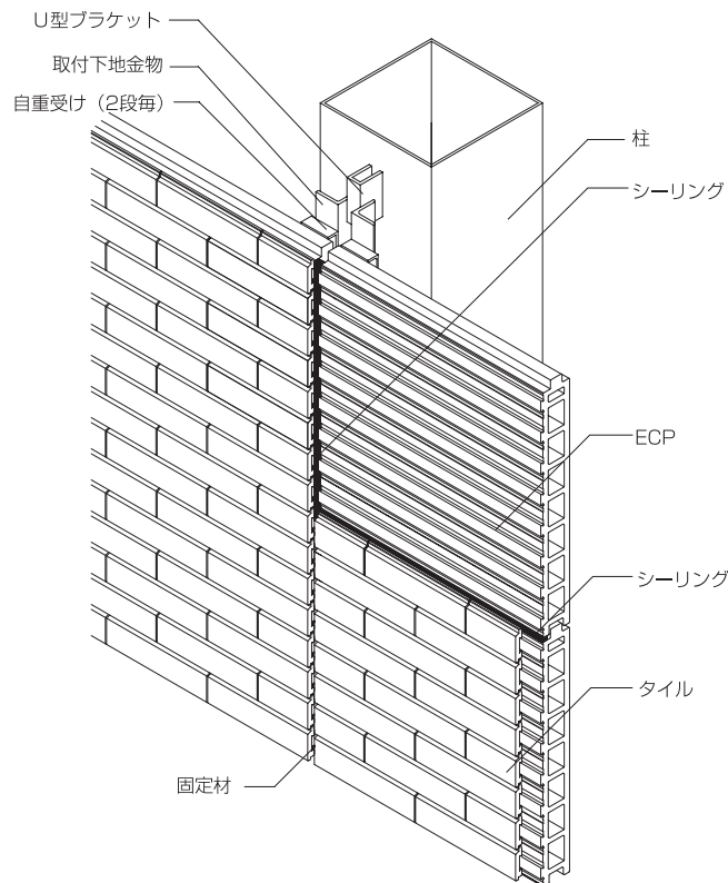
図6-6 乾式タイルパネル姿図
