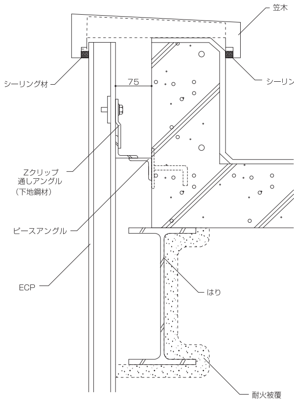
図4-10 縦張り工法上部標準詳細図
