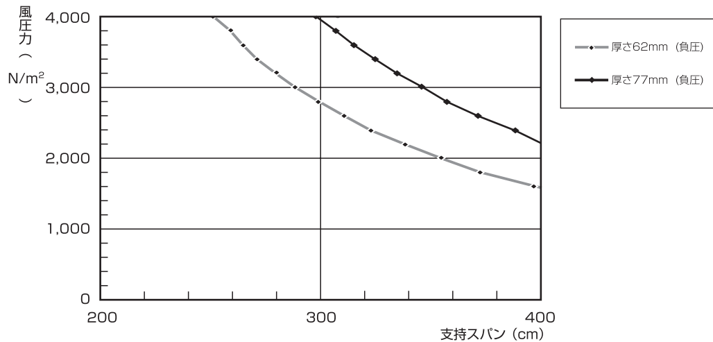
図6-3 タイル仕上げパネルの風圧と支持スパン
