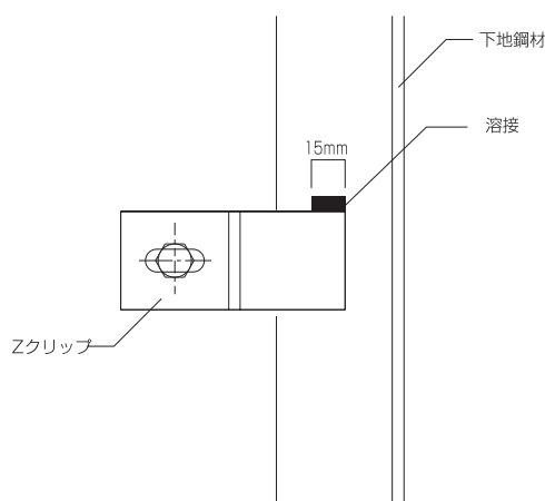
図4-16 Zクリップの取付け
