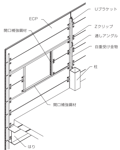
図4-2 横張り工法
