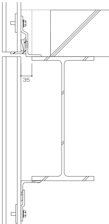
図4-4 縦張り工法
