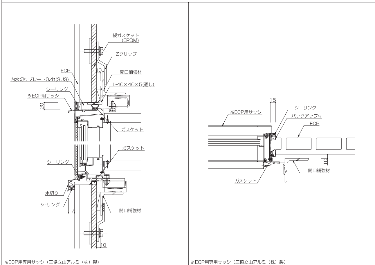
開口部垂直・水平断面詳細図
