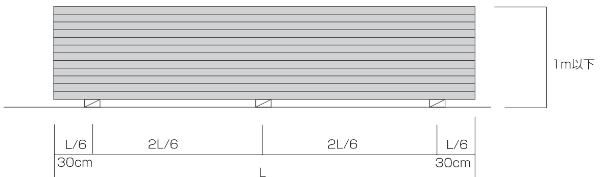
パネル長さが4mを超える場合
