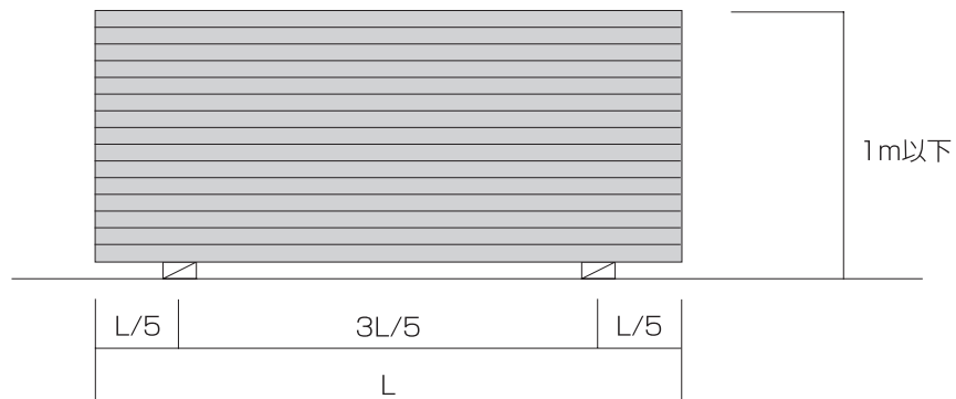
パネル長さが4m以下の場合
