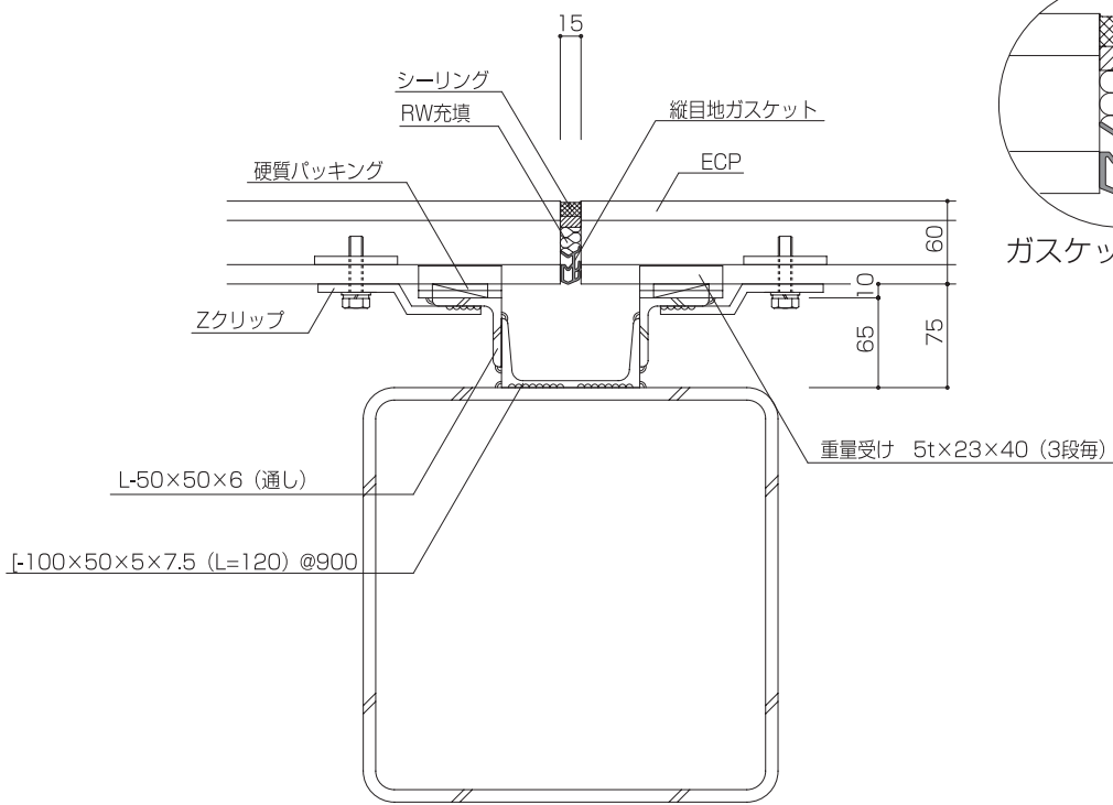
水平断面図
