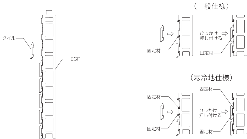
図6-4 乾式タイルパネル断面図
